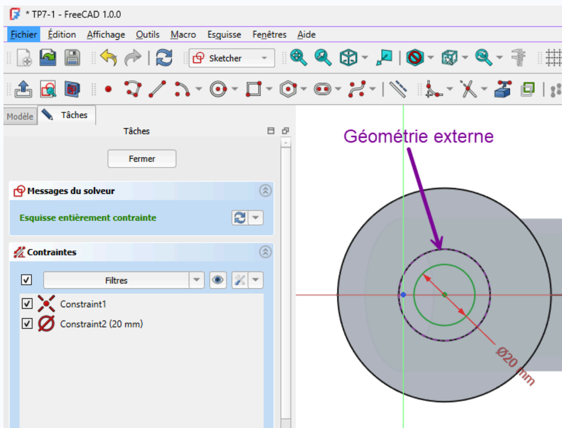
Cavités : esquisse sur la face en bout du 2 nd cylindre
