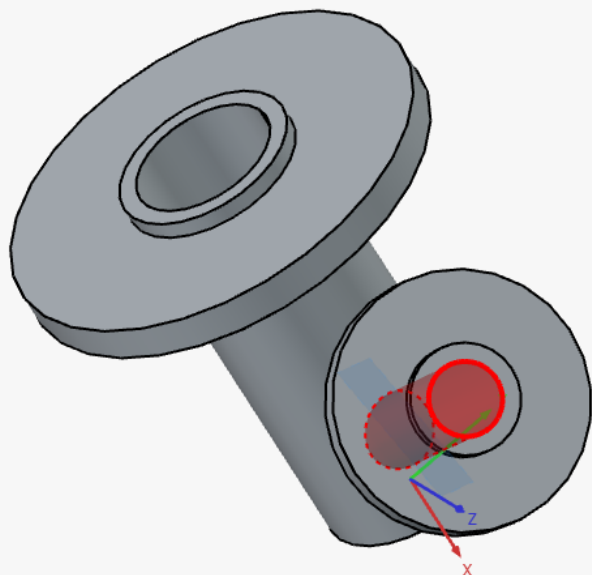
Création de la cavité sur le 2 nd cylindre
