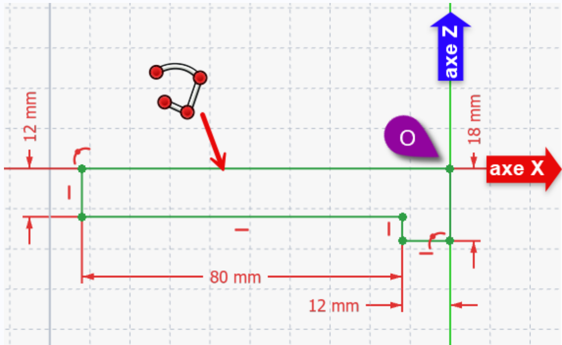
1 ère esquisse
